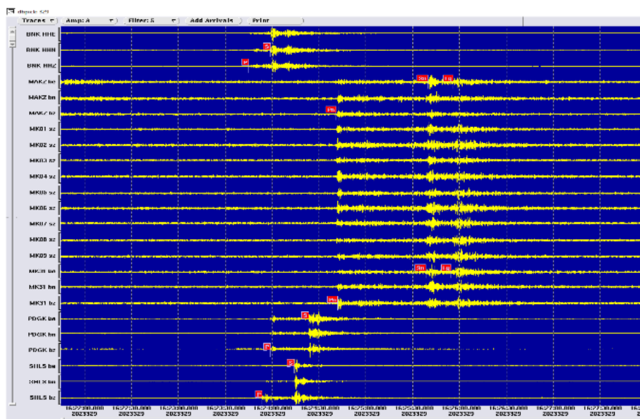
Рисунок 14. Записи ледникового землетрясения станциями ближней зоны и группой Маканчи, энергетический класс 6,1
