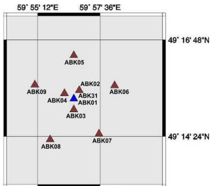
Рис. 5. Схема расположения элементов сейсмической группы «Амбулак»
