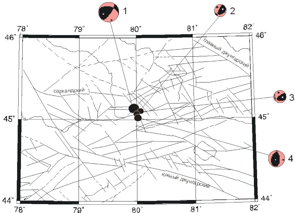
Рис. 8. Стереогаммы механизмов очагов землетрясения 27 октября с K_p=14.5 и его трех афтершоков в проекции нижней полусферы
