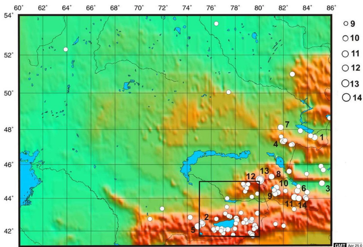
Рис. 7. Карта эпицентров землетрясений Казахстана (включен район «Северный Тянь-Шань», выделенный рамкой) с K_p \geq 8.6 за 2004 г.
