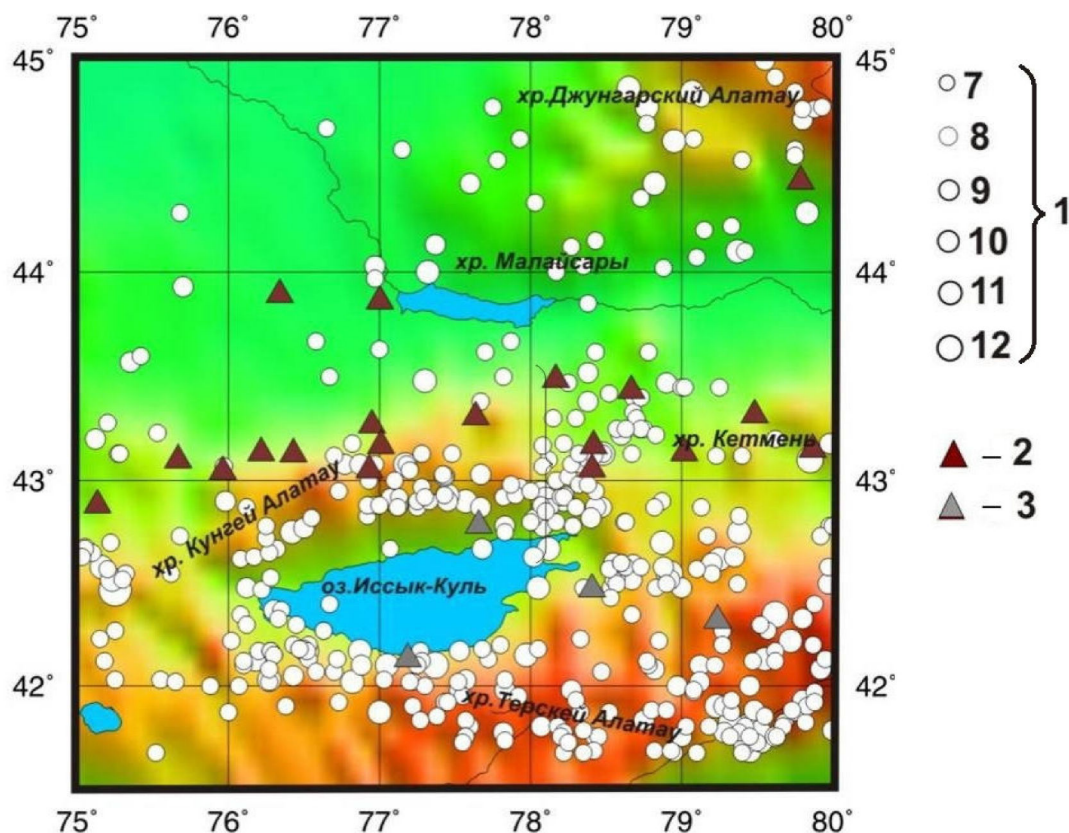
Рис. 3. Карта эпицентров землетрясений Северного Тянь-Шаня с K_p \geq 6.6 за 2004 г.
