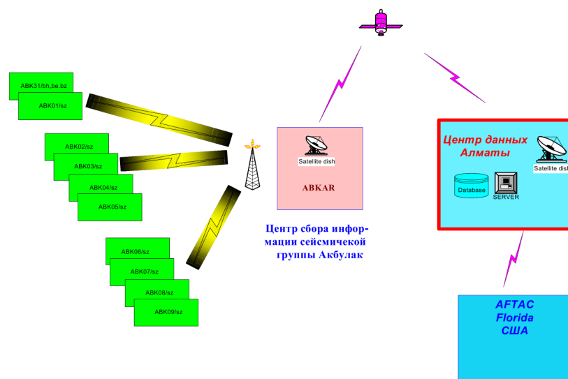
Рис. 6. Схема организации сбора и передачи данных сейсмической группы «Акбулак»
