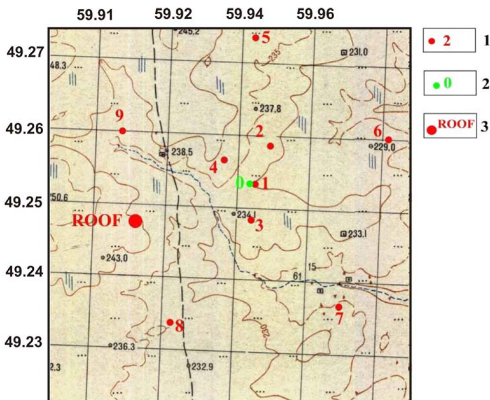
Рис. 4. Топографическая карта участка размещения сейсмической группы «Акбулак»
