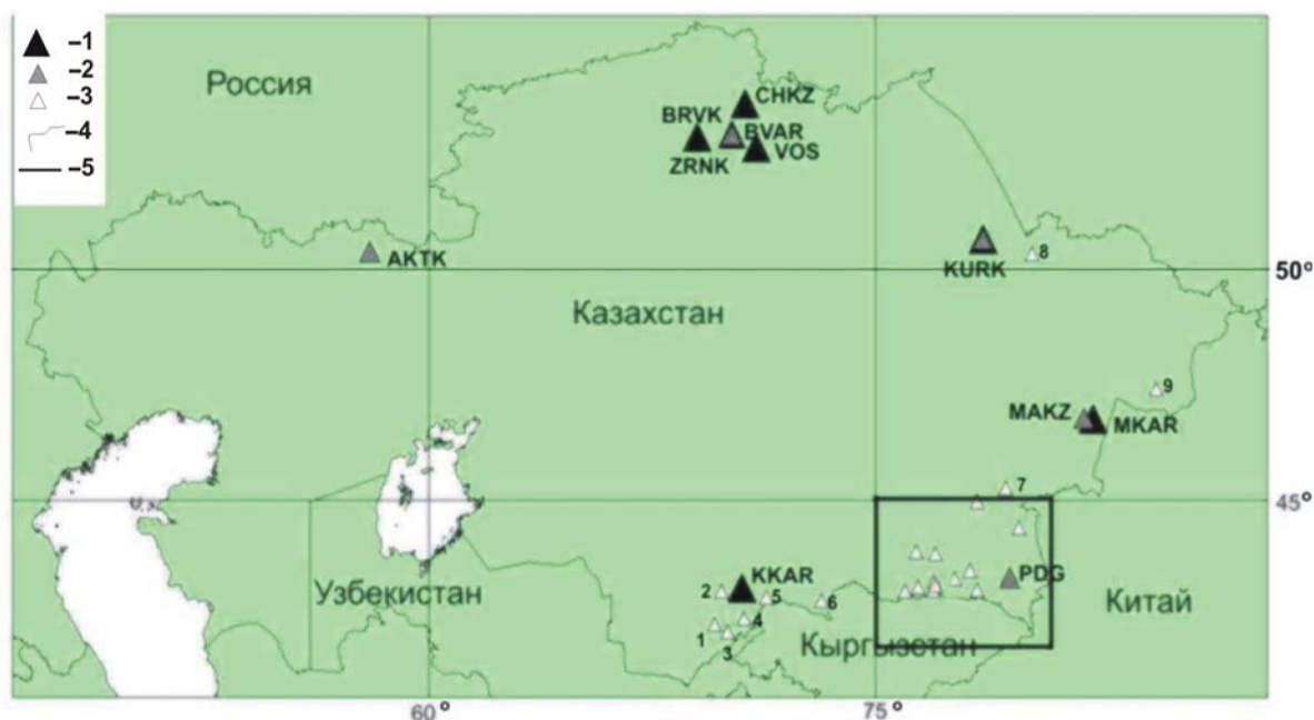
Рис. 2. Схема размещения сейсмических станций на территории Казахстана
