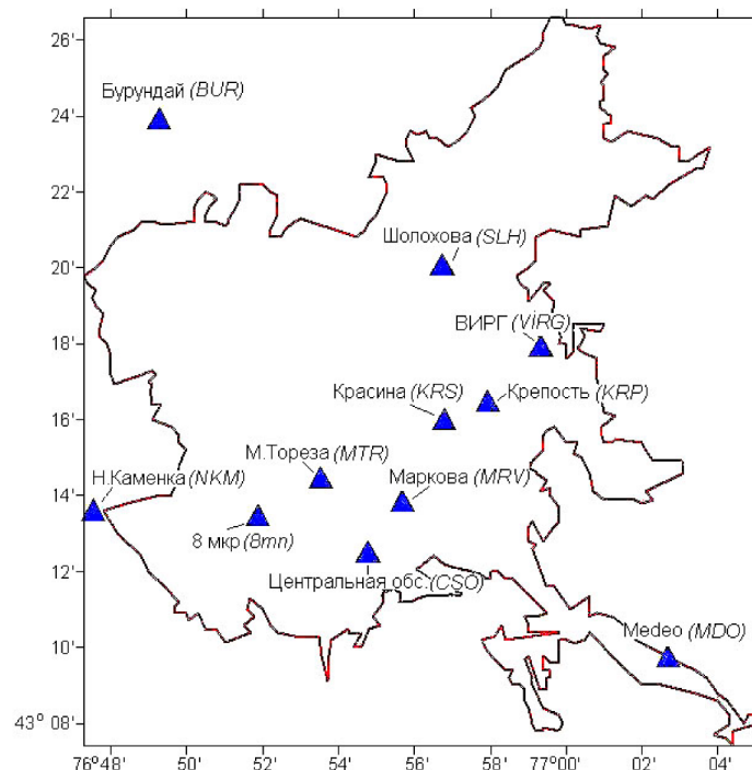
Рис. 4. Станции сети сильных движений на территории г. Алматы, записавшие землетрясение 1 декабря в 01 h 38 m с K_p=14.3
