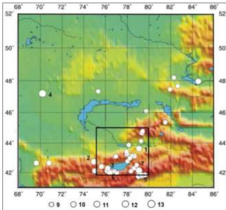
Рис. 5. Карта эпицентров землетрясений Казахстана, включая район «Северный Тянь-Шань»
