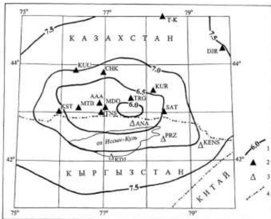
Рис. 4. Карта энергетической представительности землетрясений K^ Северного Тянь-Шаня за 2001 г.
