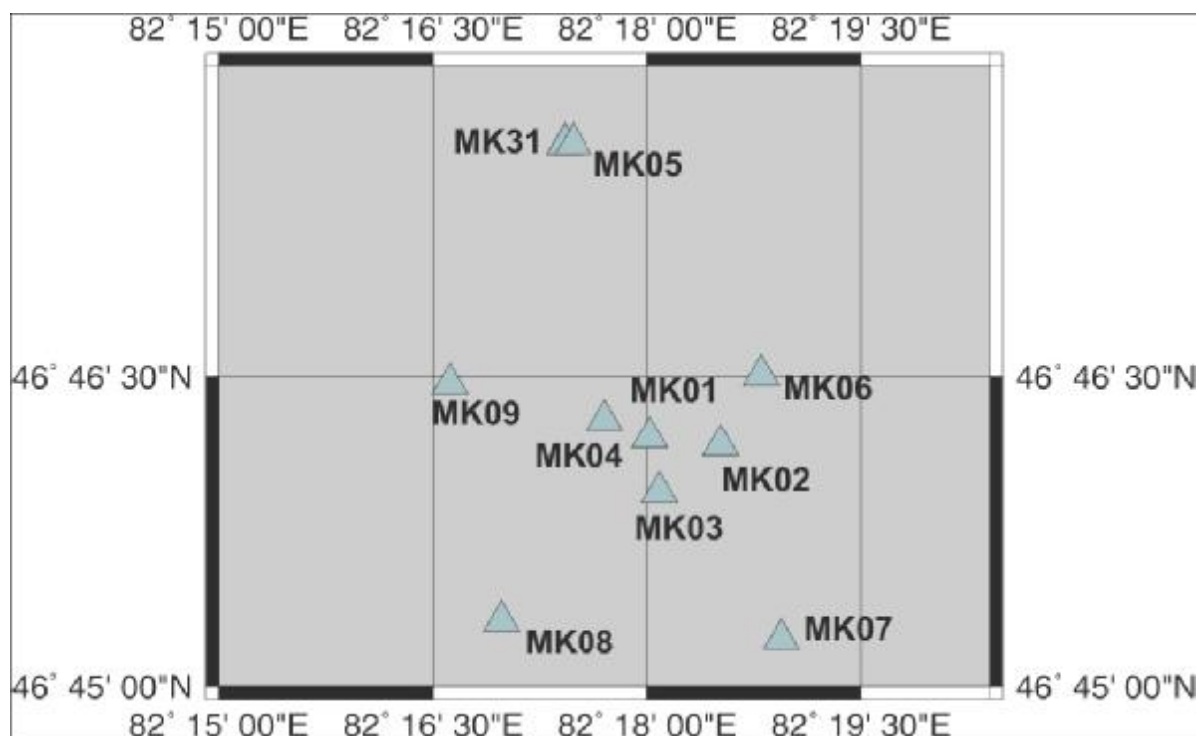
Рис. 1. Схема расположения элементов сейсмической группы «Мақанчи»
