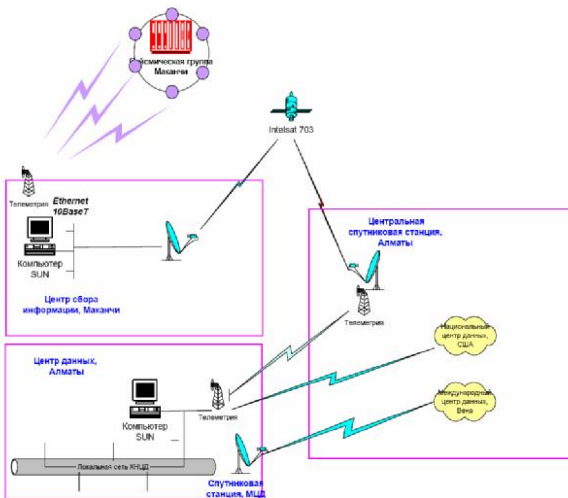
Рис. 2. Схема организации потока данных от станции «Мақанчи» в Центр данных, г. Алматы
