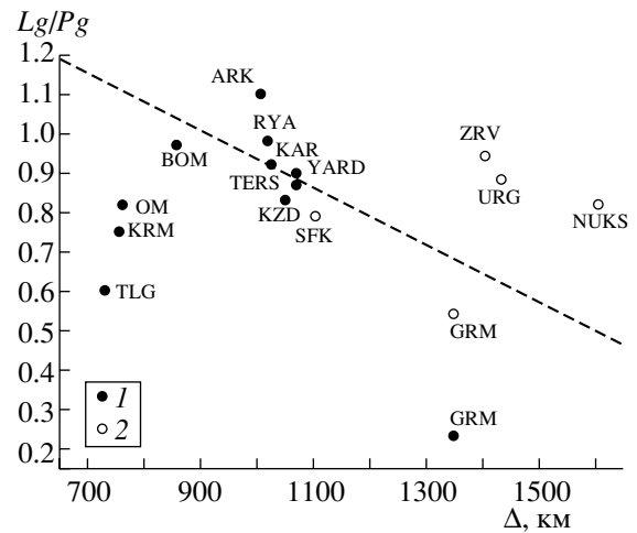
Рис. 3. Зависимость параметра Lg/Pg от эпицентрального расстояния. 1 – данные за 1965–1966 гг., 2 – за 1970–1971 гг. Штриховая линия – средняя зависимость для районов Тянь-Шаня и Туранской плиты.
