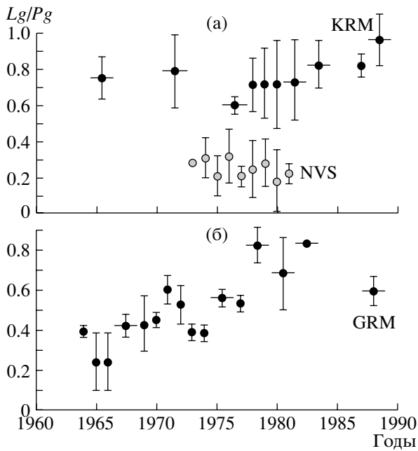
Рис. 2. Временные вариации параметра Lg/Pg . а – ст. NVS и KRM, б – ст. GRM. Показаны средние значения, доверительные интервалы и интервалы осреднения (во всех остальных случаях они равны 1 году). В двух случаях, когда не показаны доверительные интервалы, они не превышают размеров значка.
